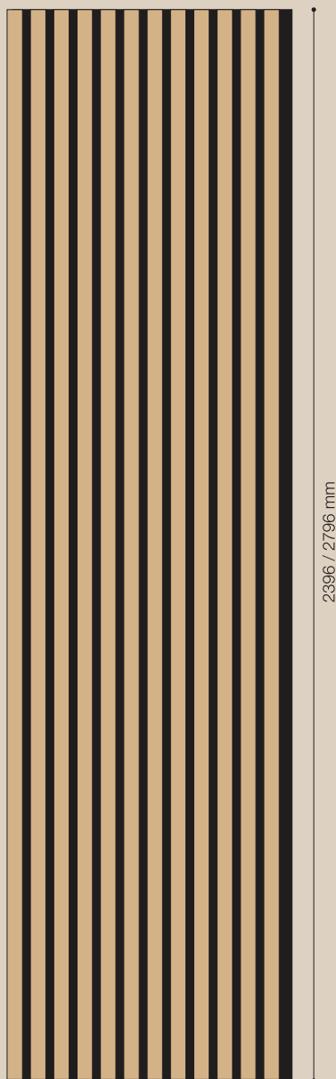
Vildi riba 9 x 38 x 2400 / 2800 mm
