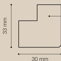
Otsa vormimine 33 x 30 x 2400 / 2800 mm
